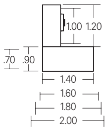
Conjunto ejecutivo, escritorio + lateral con pedestal + mamparas.
