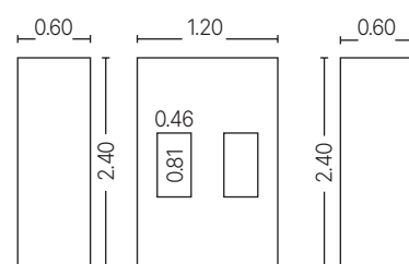
Benching completo + cajonera doble y/o pedestal móvil.
