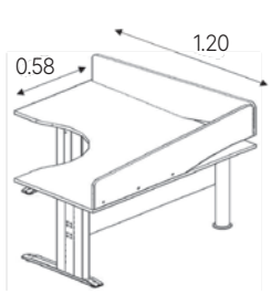
Cruceta operativa, esquineros con mampara + pedestal fijo + cubierta conector.
