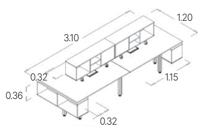
Benching 4 y 2 usuarios + libreros laterales suspendidos + libreros sobre cubierta
