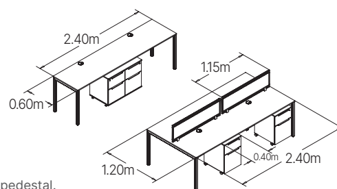
Benching doble con pedestal.
