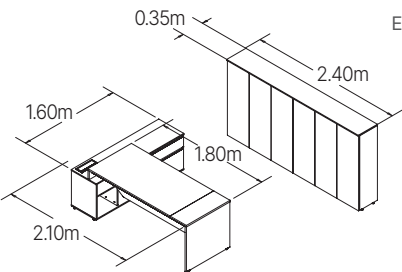
Escritorio sobre credenza con libreros medios.
