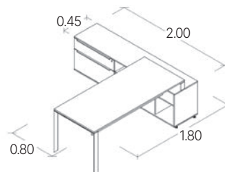
Conjunto ejecutivo; escritorio + credenza + libreros inferiores, conjunto ejecutivo; escritorio + lateral con pedestal + mamparas.
