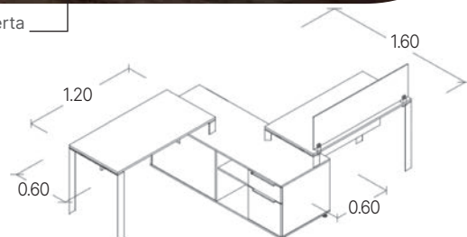
Benching 1 usuario + credenza doble vista + mamparas configuración en zeta.
