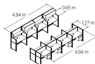
Estación en H.
