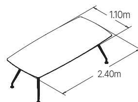
Mesa de consejo de piedra fenolica y estructura de aluminio pulido.
